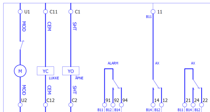
Koblingskjema
